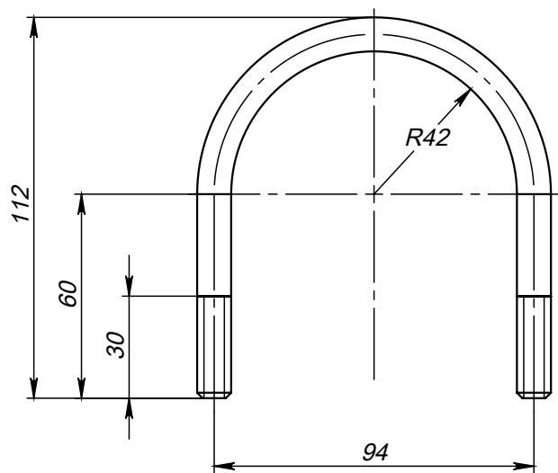
Поз.4 (Хомут)
